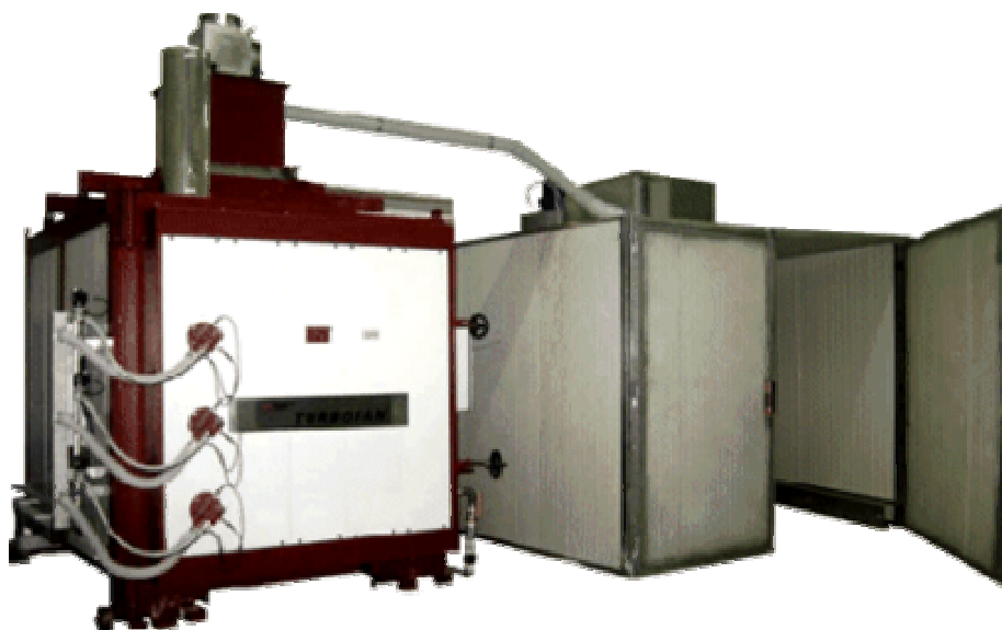
Esempio di forno turbo gas, da 2 mc collegato all'essicatoio per il recupero del calore.
